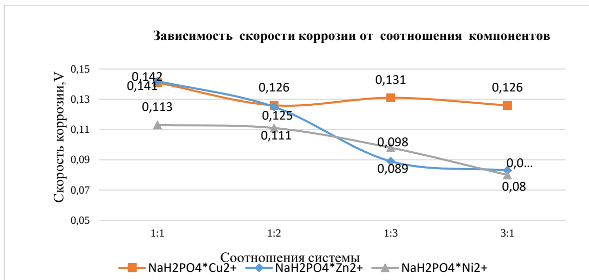
Рисунок 2 – Зависимость скорости коррозии от природы фосфата при различном соотношении
