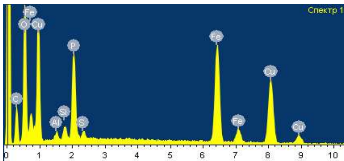
Рисунок 4 - Спектральная шкала элементов для коррозионного отложения композиции \text{NaH}_2\text{PO}_4 \cdot \text{Ni}^{2+} в соотношении 3:1
