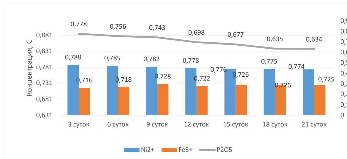
Рисунок 1 –Изменение концентрации иона модификатора никеля, железа, фосфата от времени для системы дигидрофосфата натрия
