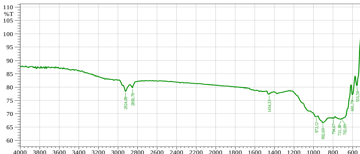
Рисунок 3 – Анализ коррозионного отложения дигидрофосфата натрия \text{NaH}_2\text{PO}_4
