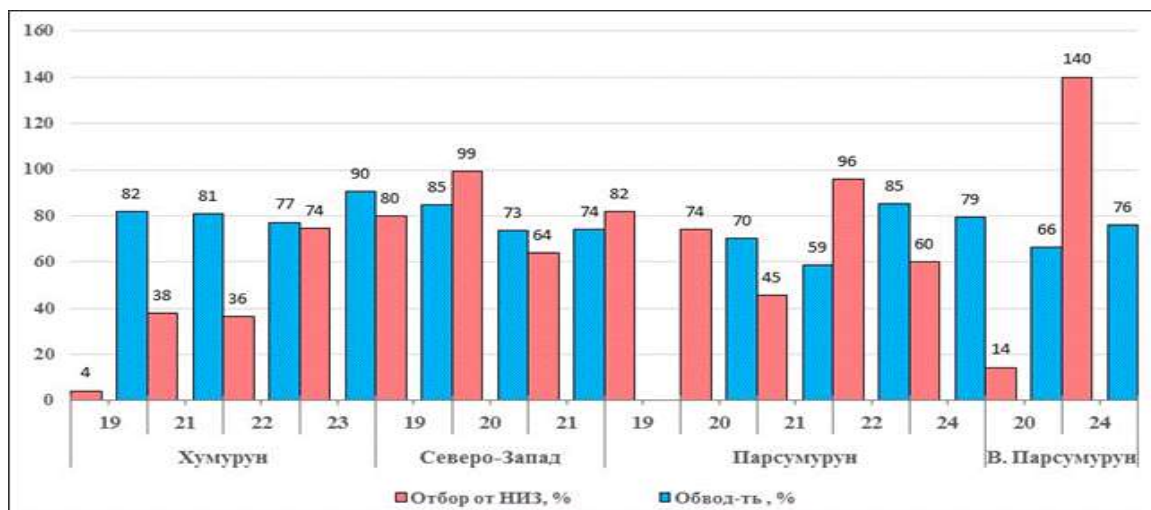
Рисунок 2 - Обводненность и отбор от утвержденных извлекаемых запасов по горизонтам
