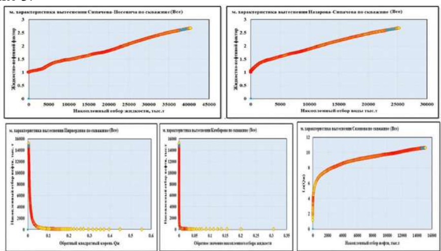
Рисунок 3-Характеристика вытеснения по разным методам по 19-24 горизонтам месторождения
